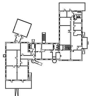
Winkelförmiger Grundriss
